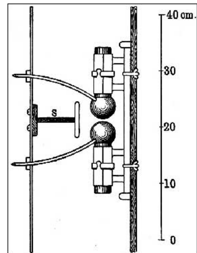
Sender-Kugelfunkenstrecke
