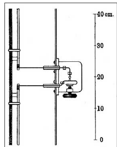
Resonator-Funkenstrecke mit Mikrometerschraube.
