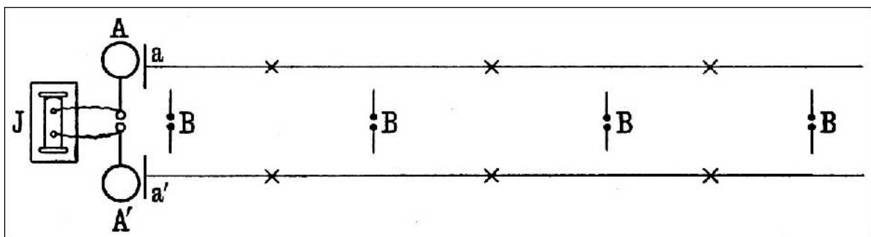
Angeregte Lecherleitung mit Spannungsbäuchen und -knoten zur Wellenlängen-Bestimmung.
