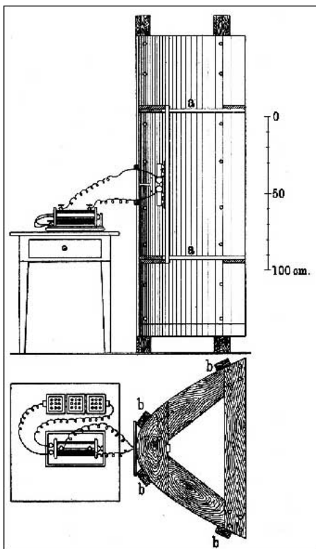
Parabolspiegel mit der Sender-Funkstrecke im Brennpunkt.
