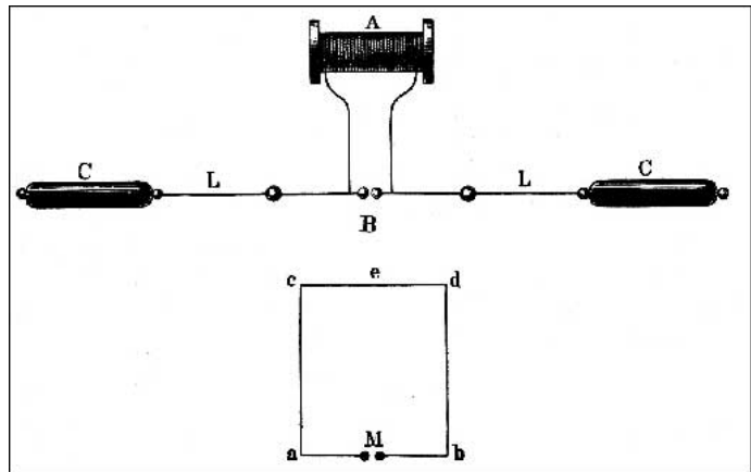
Hertz'sche Versuchsanordnung mit Funkeninduktor A, Luftleiter L mit Sender-Funkenstrecke B und Resonanzkreis mit Kontroll-Funkenstrecke M.
